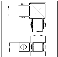
klembeugel hoekpaal
