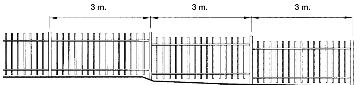
hekverloop verspringen
